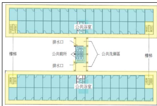
「H」型徙置大廈的平面圖
